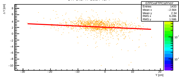
GTPCvsFTPC1 \Delta Y
