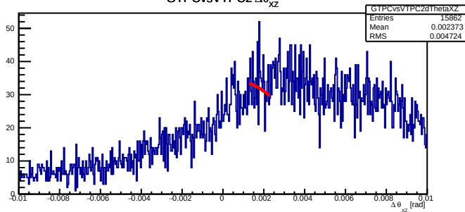
GTPCvsVTPC2 \Delta\theta_{xz}
