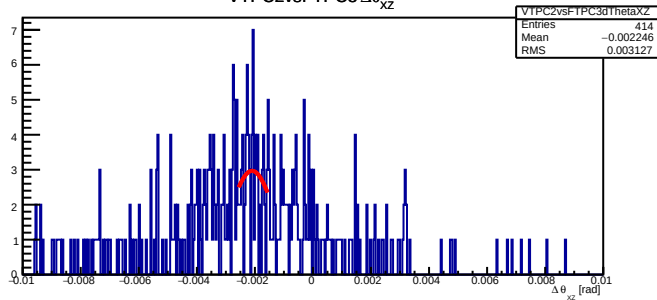
VTPC2vsFTPC3 \Delta\theta_{xz}
