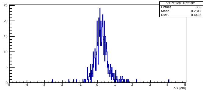
VTPC1vsFTPC1 \Delta Y
