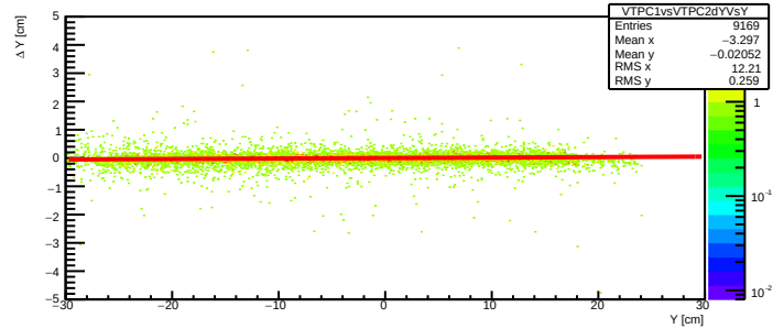
VTPC1vsVTPC2 \Delta Y
