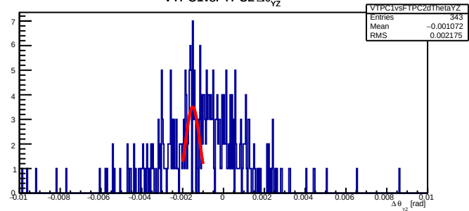
VTPC1vsFTPC2 \Delta\theta_{yz}
