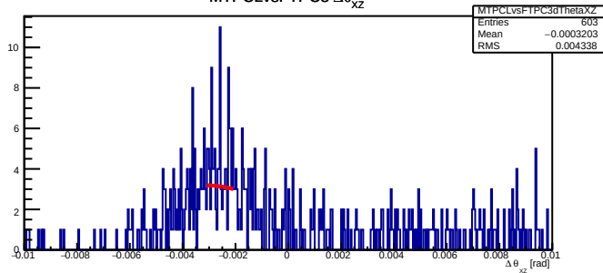
MTPCLvsFTPC3 \Delta\theta_{xz}
