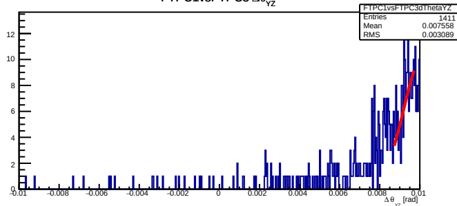
FTPc1vsFTPc3 \Delta\theta_{yz}
