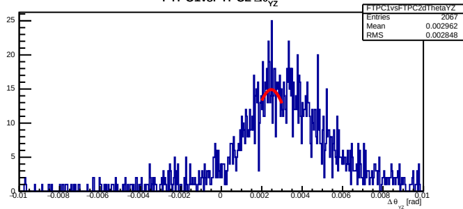
FTPC1vsFTPC2 \Delta\theta_{yz}
