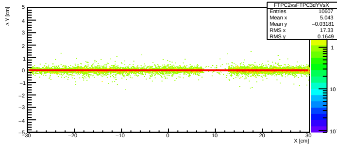
FTPC2vsFTPC3 \Delta Y vs. X
