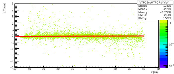
VTPC2vsMTPCR \Delta Y
