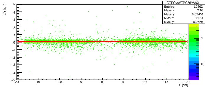
GTPCvsVTPC2 \Delta Y vs. X
