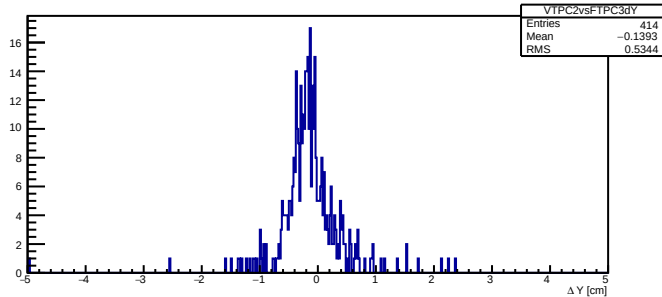
VTPC2vsFTPC3 \Delta Y
