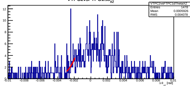
VTPC2vsFTPC1 \Delta\theta_{xz}
