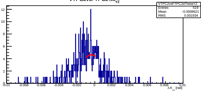
VTPC2vsFTPC2 \Delta\theta_{yz}
