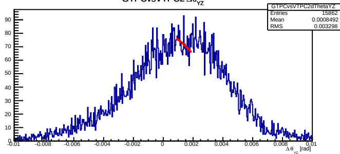
GTPCvsVTPC2 \Delta\theta_{yz}
