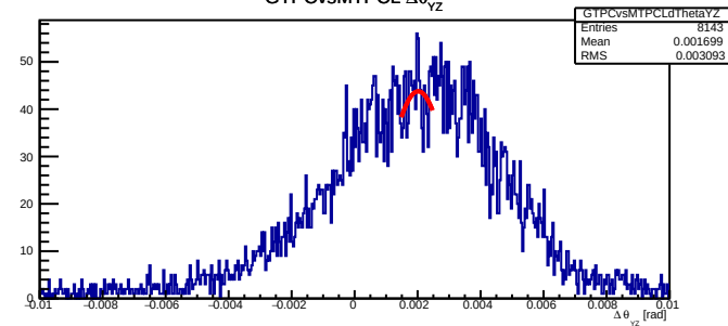
GTPCvsMTPCL \Delta\theta_{yz}
