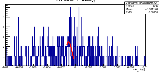
VTPC1vsFTPC1 \Delta\theta_{xz}
