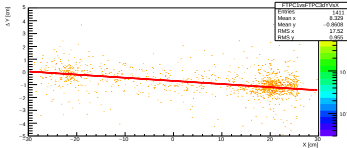
FTPc1vsFTPc3 \Delta Y vs. X
