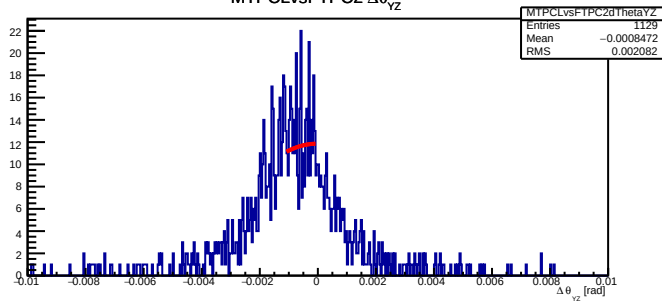
MTPCLvsFTPC2 \Delta\theta_{yz}
