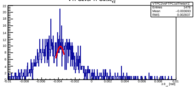
VTPC2vsFTPC1 \Delta\theta_{yz}
