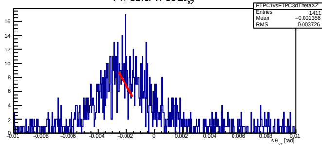
FTPc1vsFTPc3 \Delta\theta_{xz}
