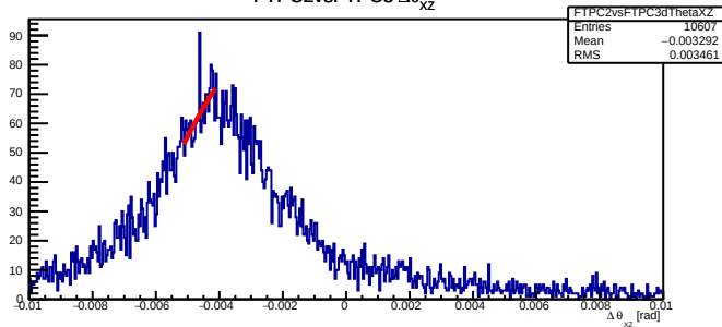
FTPC2vsFTPC3 \Delta\theta_{xz}
