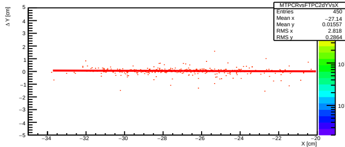
MTPCRvsFTPC2 \Delta Y vs. X
