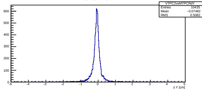
VTPC2vsMTPCR \Delta Y
