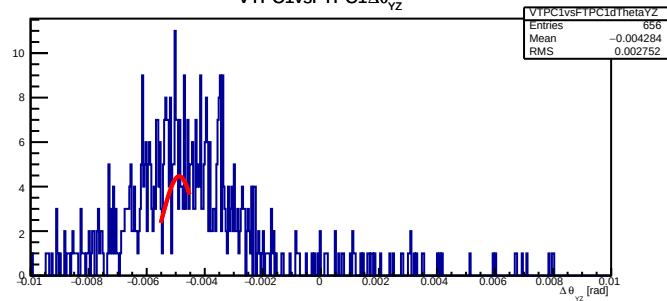
VTPC1vsFTPC1 \Delta\theta_{yz}
