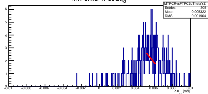
MTPCRvsFTPC3 \Delta\theta_{yz}
