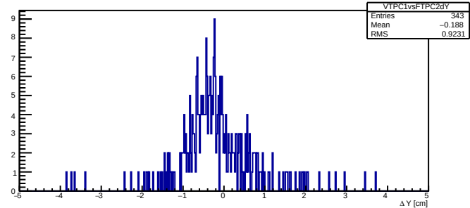
VTPC1vsFTPC2 \Delta Y
