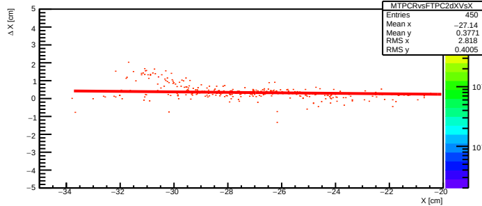
MTPCRvsFTPC2 \Delta X vs. X
