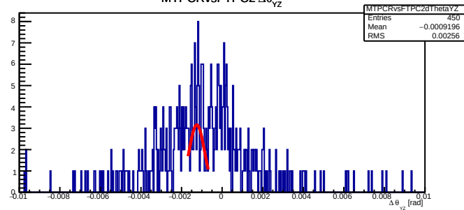
MTPCRvsFTPC2 \Delta\theta_{yz}
