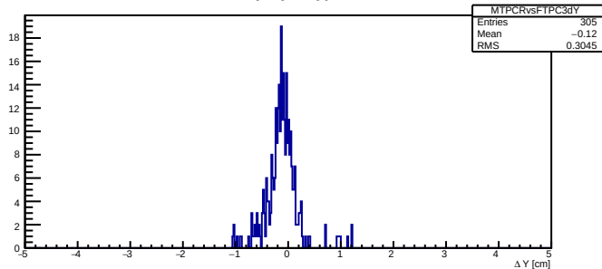
MTPCRvsFTPC3 \Delta Y
