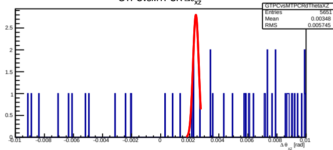
GTPCvsMTPCR \Delta\theta_{xz}
