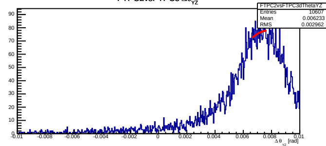
FTPC2vsFTPC3 \Delta\theta_{yz}
