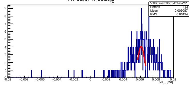
VTPC2vsFTPC3 \Delta\theta_{yz}
