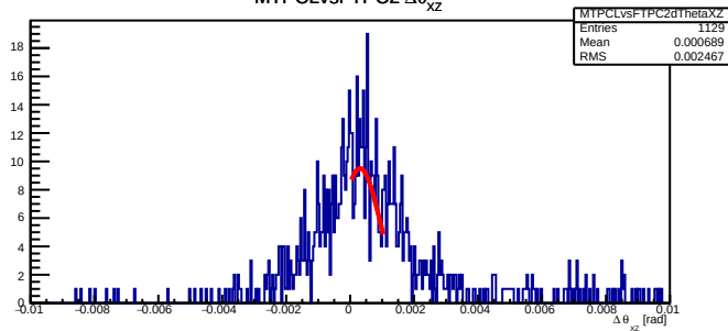
MTPCLvsFTPC2 \Delta\theta_{xz}
