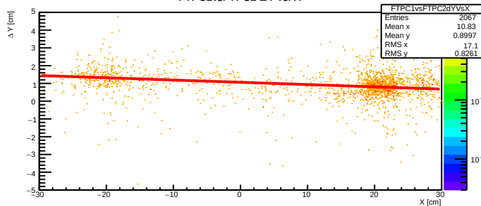
FTPC1vsFTPC2 \Delta Y vs. X
