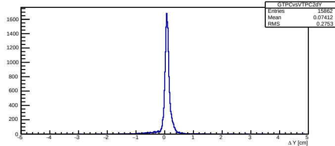
GTPCvsVTPC2 \Delta Y
