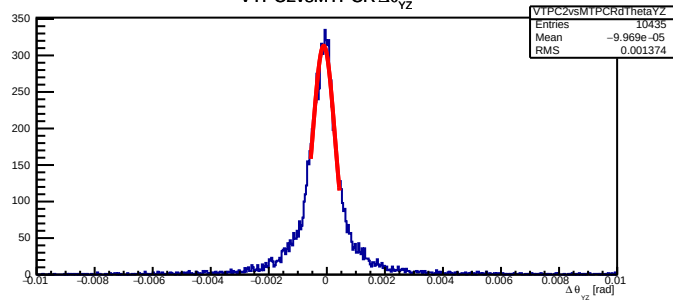
VTPC2vsMTPCR \Delta\theta_{yz}
