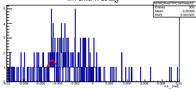
MTPCRvsFTPC3 \Delta\theta_{xz}
