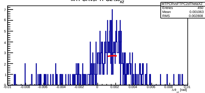
MTPCRvsFTPC2 \Delta\theta_{xz}
