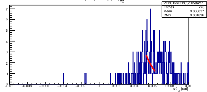
VTPC1vsFTPC3 \Delta\theta_{yz}
