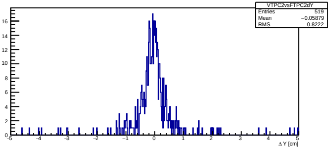
VTPC2vsFTPC2 \Delta Y
