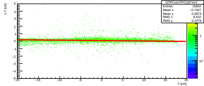
GTPCvsVTPC2 \Delta Y vs. Y
