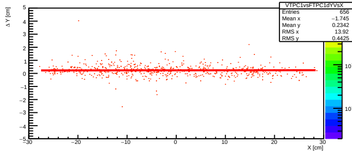
VTPC1vsFTPC1 \Delta Y vs. X
