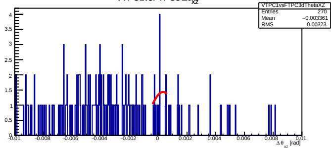
VTPC1vsFTPC3 \Delta\theta_{xz}
