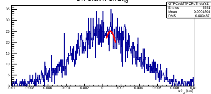
GTPCvsMTPCR \Delta\theta_{yz}
