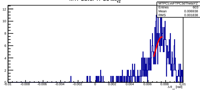
MTPCLvsFTPC3 \Delta\theta_{yz}
