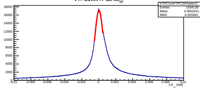
VTPC1vsVTPC2 \Delta\theta_{yz}
