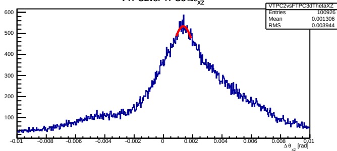
VTPC2vsFTPC3 \Delta\theta_{xz}
