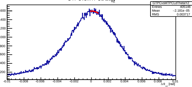
GTPCvsMTPCL \Delta\theta_{yz}
