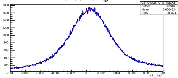
GTPCvsMTPCR \Delta\theta_{xz}
