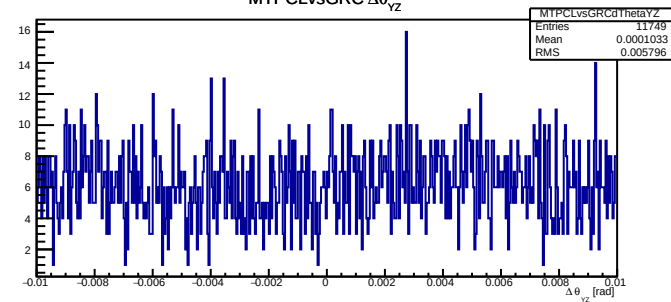
MTPCLvsGRC \Delta\theta_{yz}
