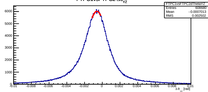
FTPC1vsFTPC2 \Delta\theta_{yz}
