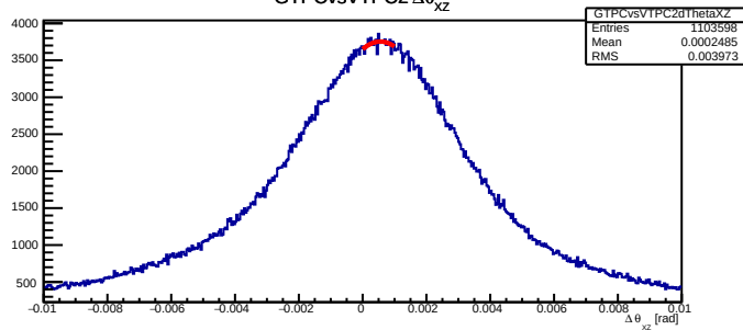
GTPCvsVTPC2 \Delta\theta_{xz}
