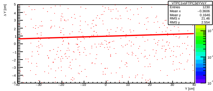
VTPC1vsFTPC3 \Delta Y vs. Y
