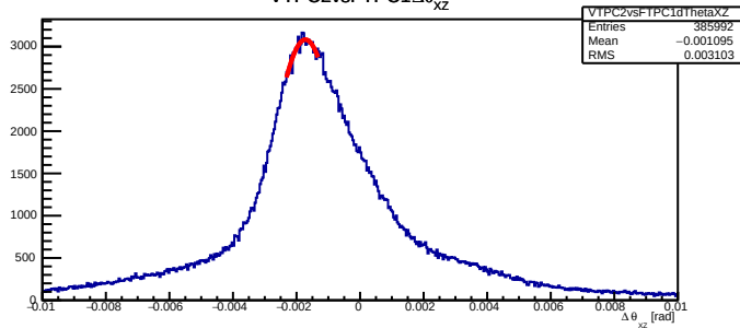
VTPC2vsFTPC1 \Delta\theta_{xz}
