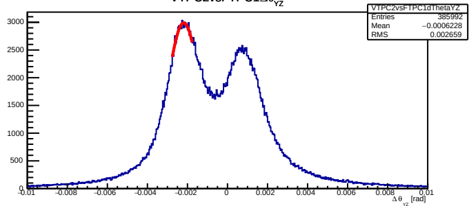
VTPC2vsFTPC1 \Delta\theta_{yz}
