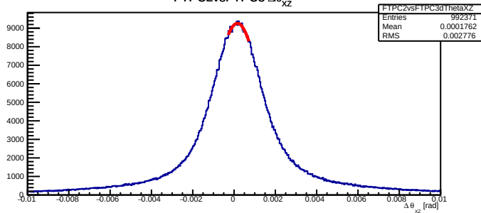
FTPC2vsFTPC3 \Delta\theta_{xz}
