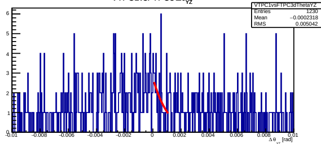
VTPC1vsFTPC3 \Delta\theta_{yz}
