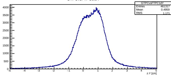
GTPCvsFTPC1 \Delta Y
