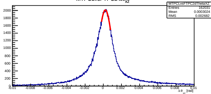
MTPCLvsFTPC2 \Delta\theta_{xz}
