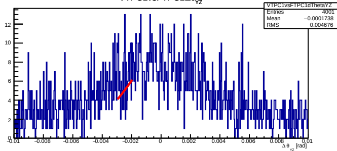
VTPC1vsFTPC1 \Delta\theta_{yz}
