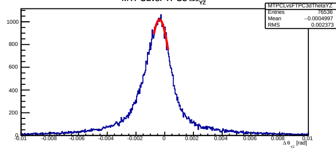
MTPCLvsFTPC3 \Delta\theta_{yz}
