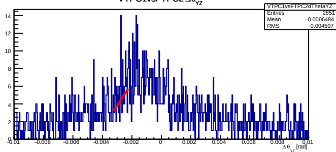
VTPC1vsFTPC2 \Delta\theta_{yz}
