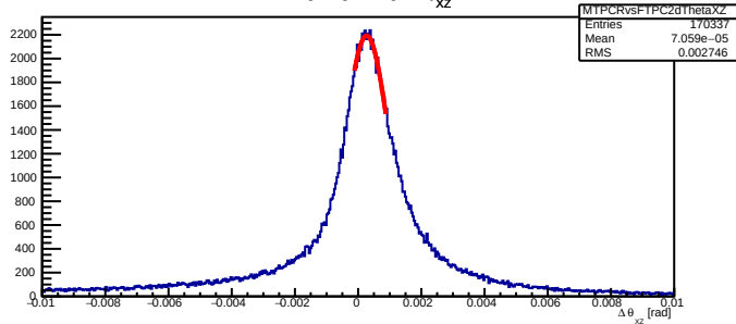
MTPCRvsFTPC2 \Delta\theta_{xz}
