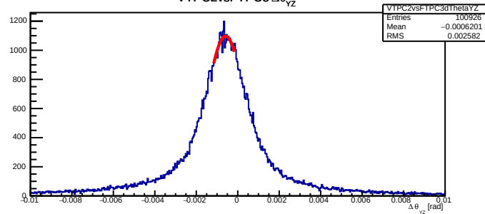
VTPC2vsFTPC3 \Delta\theta_{yz}
