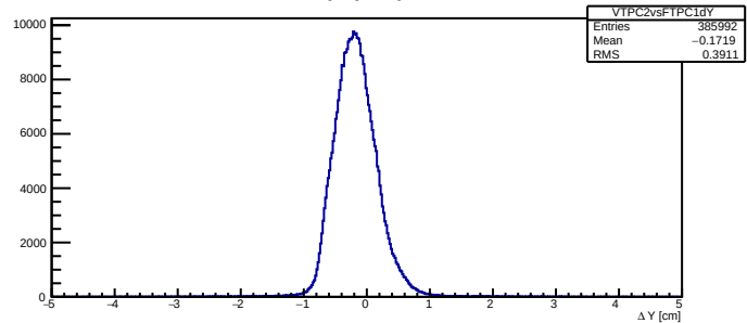
VTPC2vsFTPC1 \Delta Y
