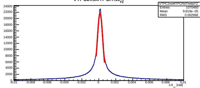
VTPC2vsMTPCR \Delta\theta_{yz}
