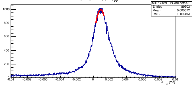
MTPCRvsFTPC3 \Delta\theta_{xz}
