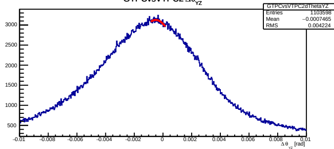
GTPCvsVTPC2 \Delta\theta_{yz}
