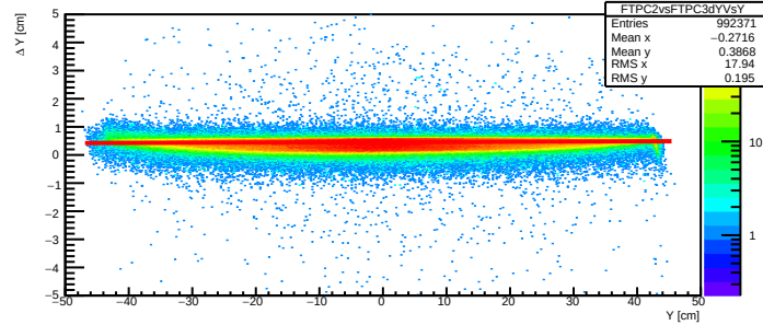
FTPC2vsFTPC3 \Delta Y
