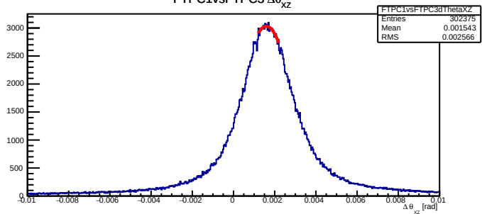
FTPC1vsFTPC3 \Delta\theta_{xz}
