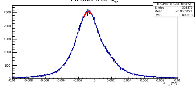
FTPC1vsFTPC3 \Delta\theta_{yz}
