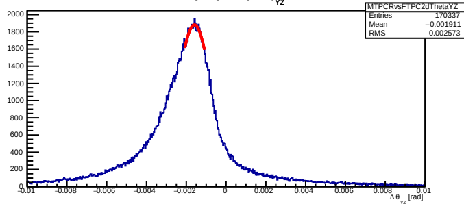
MTPCRvsFTPC2 \Delta\theta_{yz}
