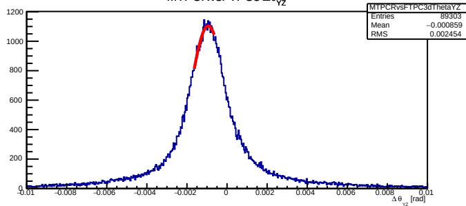
MTPCRvsFTPC3 \Delta\theta_{yz}
