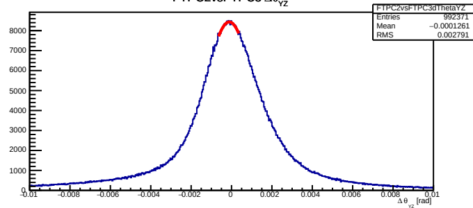
FTPC2vsFTPC3 \Delta\theta_{yz}
