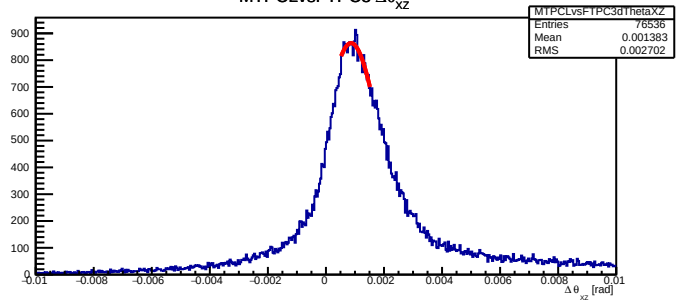
MTPCLvsFTPC3 \Delta\theta_{xz}
