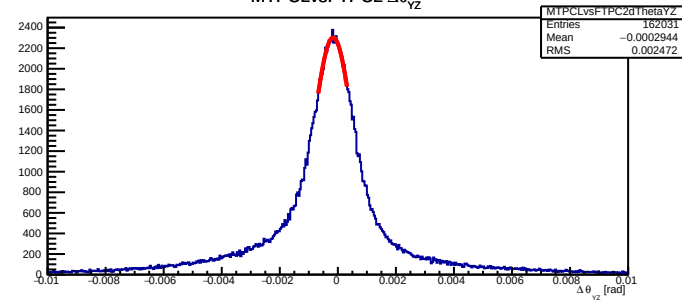
MTPCLvsFTPC2 \Delta\theta_{yz}
