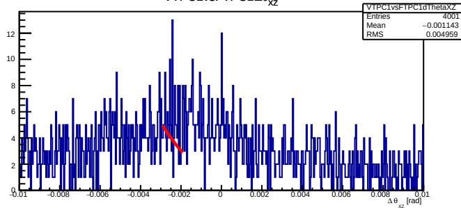
VTPC1vsFTPC1 \Delta\theta_{xz}
