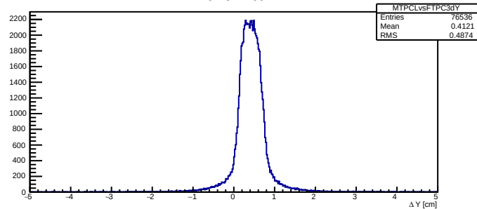
MTPCLvsFTPC3 \Delta Y
