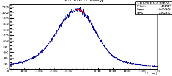
GTPCvsFTPC1 \Delta\theta_{xz}
