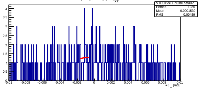
VTPC1vsFTPC3 \Delta\theta_{xz}
