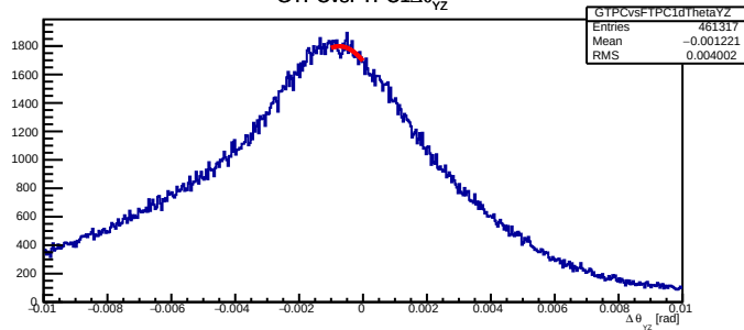
GTPCvsFTPC1 \Delta\theta_{yz}
